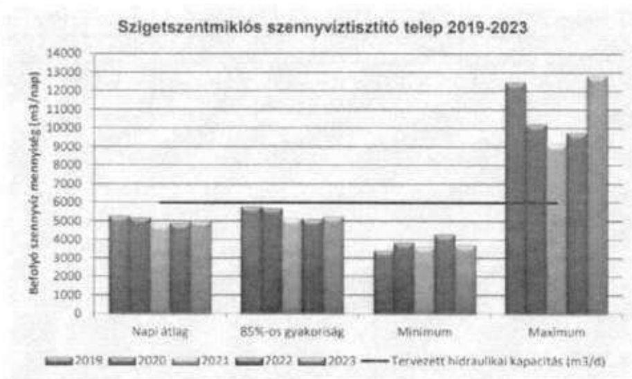
11. ábra: Szennyvíztisztító telepre befolyó szennyvízmennyiség (2019-2023)
