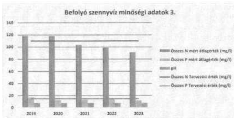
15. ábra: Befolyó szennyvíz minőségi adatok –összes N, összes P, pH (2019-2023)
