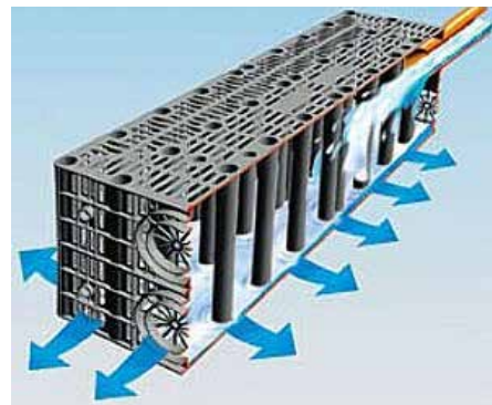
Föld alá helyezhető szikkasztóblokk
